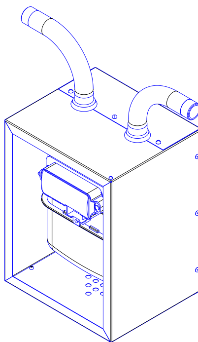
Рис. 13 Розміщення лічильника газу в шафі захисній (дверцята шафи умовно не показані).
