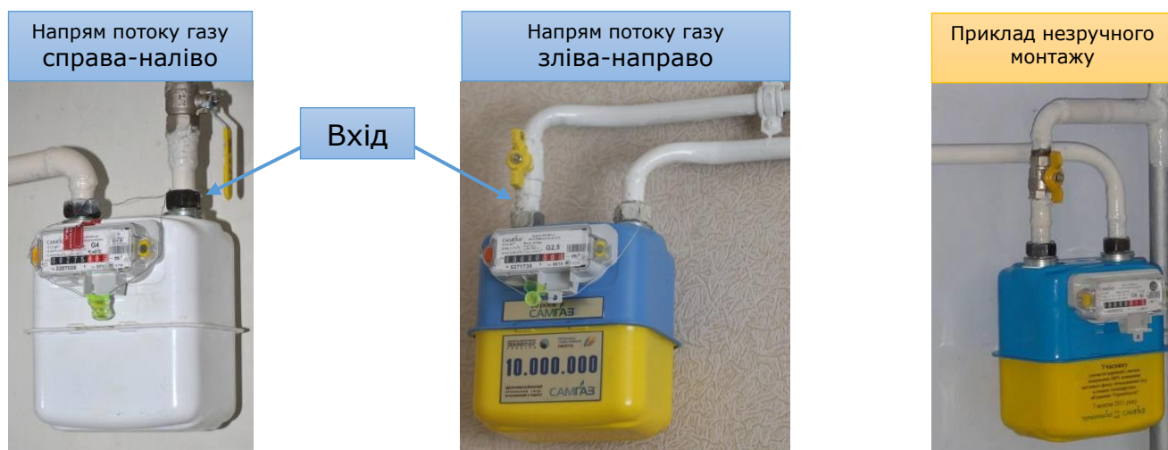
Рис. 8 Приклади монтажу лічильників газу
